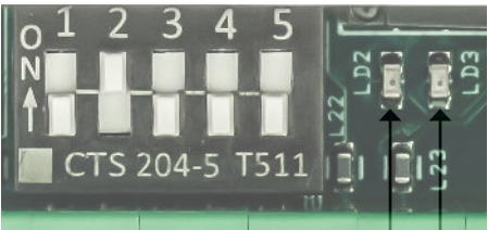
DIP-Schalter
