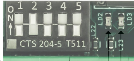
Commutateur DIP
