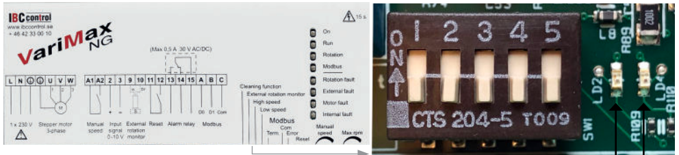
DIP-valintakytkin
